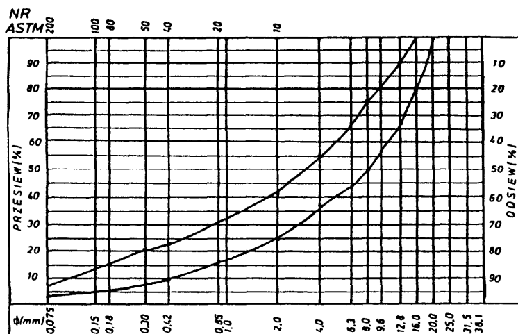
Rys. 6. Krzywe graniczne uziarnienia mieszanki mineralnej 0÷20 mm do warstwy wiążącej, wyrównawczej i wzmacniającej z mieszanki mineralno – asfaltowej dla KR 3-6
