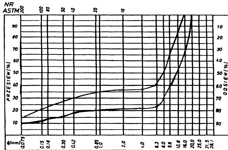
Rys. 3. Krzywe graniczne uziarnienia mieszanki mineralnej 0+16 mm do warstwy ściernalnej z mieszanki mineralno – asfaltowej dla KR 3-6
