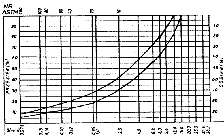
Rys. 4. Krzywe graniczne uziarnienia mieszanki mineralnej 0÷12,8 mm do warstwy ścieralnej z mieszanki mineralno – asfaltowej dla KR 3-6
