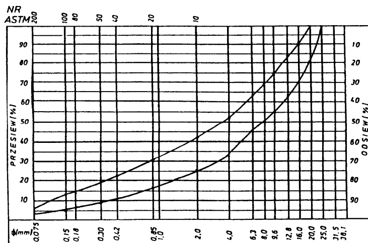
Rys. 5. Krzywe graniczne uziarnienia mieszanki mineralnej 0÷25 mm do warstwy wiążącej z mieszanki mineralno – asfaltowej dla KR 3-6
