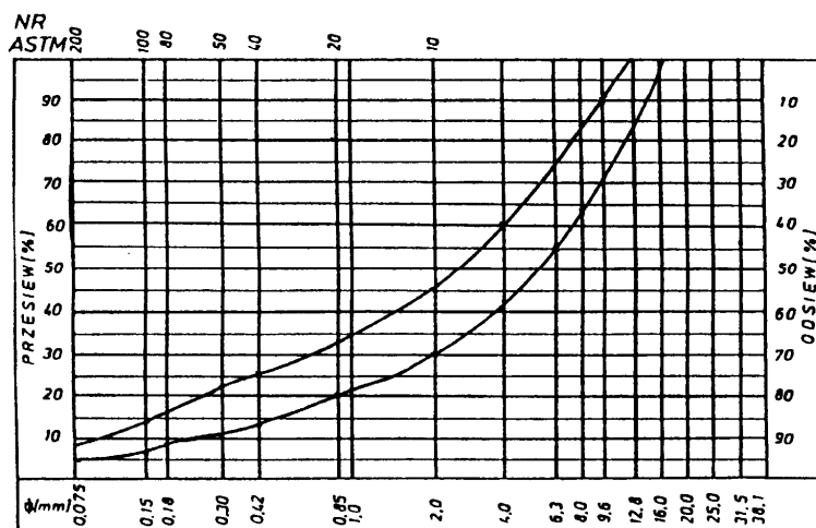
Rys. 7. Krzywe graniczne uziarnienia mieszanki mineralnej 0÷16 mm do warstwy wiążącej, wyrównawczej i wzmacniającej z mieszanki mineralno – asfaltowej dla KR 3-6.
